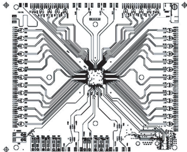
Figure 7-4. Top Layer
